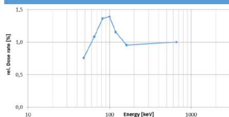
プラスチックシンチレータ エネルギー特性
