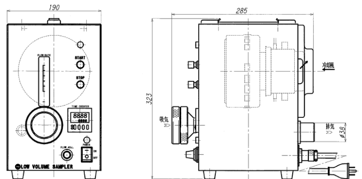
可変流量型ダストサンプラ 図面
