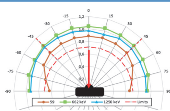
プラスチックシンチレータ 方向特性
